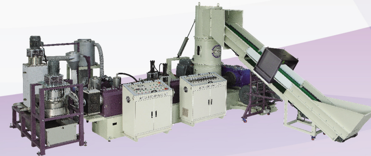
CKR-series maquina de reciclaje 3 en 1
