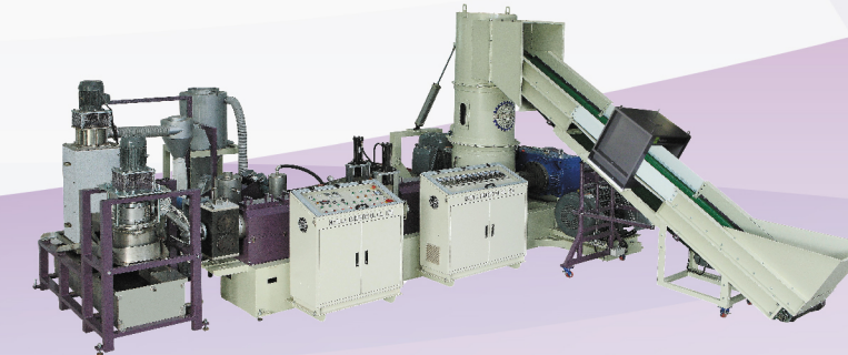
CKR-série Machine de recyclage 3 en 1 pour film plastique
