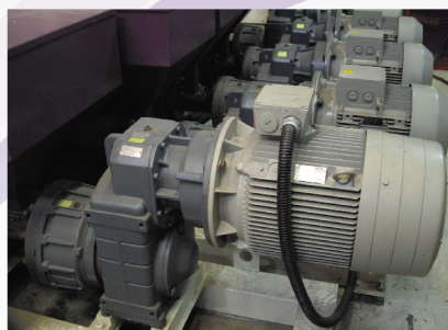
Boîte de vitesse allemande entraînement direct
