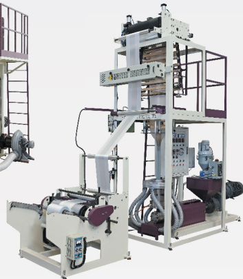
Máquina para HDPE/LDPE
