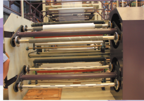
آلة مهب فيلم 3 طبقات
