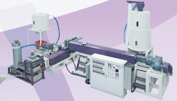
آلة اعادة تدوير البلاستيك على مرحلتين CKR-series
