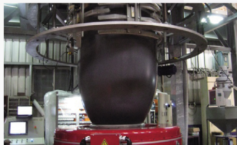
Anillo de aire automático para control del grosor
